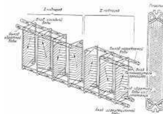
Рис. 3. Схема компоновки водоподогревателей ( и (( подогрева в одну установку с противоточным движением воды
