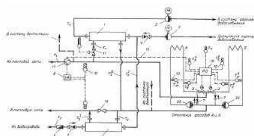
Рис. 6. Двухступенчатая схема присоединения водоподогревателей горячего водоснабжения в ИТП с зависимым присоединением систем отопления и пофасадным автоматическим регулированием расхода теплоты на отопление 1—25—см. рис. 1 — 4
