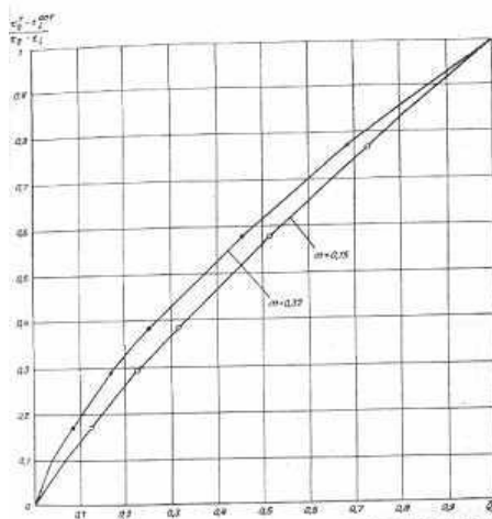
Рис. 3. Графики изменения температурного критерия системы отопления по температуре воды в обратном трубопроводе \left(\frac{\tau_2 - t_i^{opt}}{\tau_2 - t_i}\right) при постоянной циркуляции воды в системе
