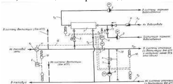
Рис. 1. Одноступенчатая система присоединения водоподогревателей горячего водоснабжения с автоматическим регулированием расхода теплоты на отопление и независимым присоединением систем отопления в ЦТП и ИТП
