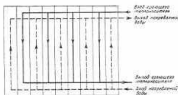
Рис. 1. Симметричная компоновка пластинчатого водоподогревателя, обозначение Сх 4/5
