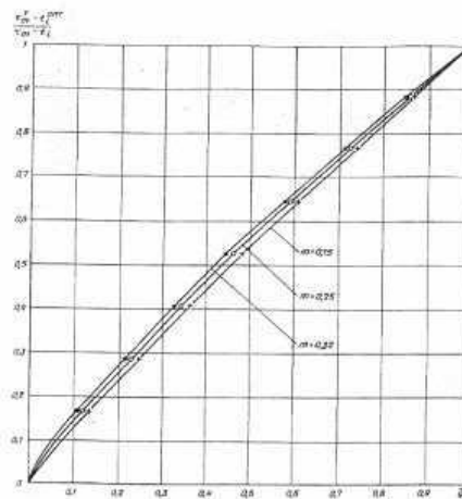
Рис. 2. Графики изменения температурного критерия системы отопления по температуре воды в подающем трубопроводе — \left(\frac{t_{01}^r - t_1^{m1}}{t_{01}^r - t_1}\right) для различных значений показателя степени m и при постоянной циркуляции теплоносителя в системе
