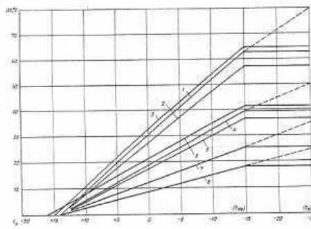
Рис. 6. Графики изменения разности температуры воды в подающем и обратном трубопроводах системы отопления ( t в зависимости от t_n )
