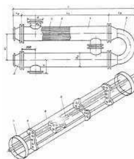
Рис. 2 Конструктивные размеры водоподогревателя
