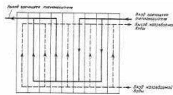
Рис. 2. Несимметричная компоновка пластинчатого водоподогревателя, обозначение Сх (2 + 2)/5
